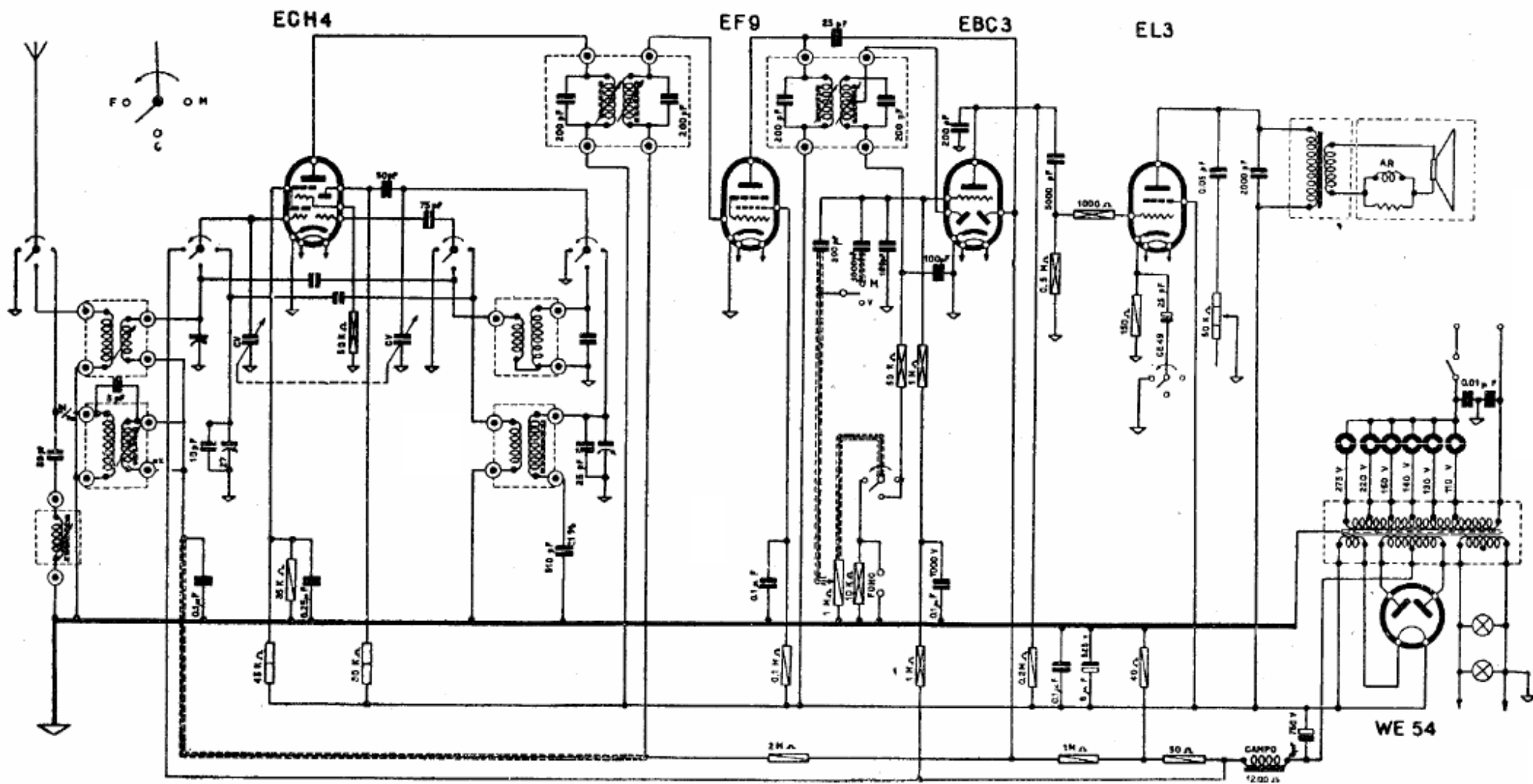
VOCE DEL PADRONE - Mod. 579 - Telaio 79.1 - Gamma onde medie da 192 a 580 m. Gamma onde corte da 16 a 60 m. Media frequenza: 465 kc/s. Potenza d'uscita: 3 W circa. Ohm eccitazione: 1200. Sintonia serie sintorapida. Produzione 1945-46.
